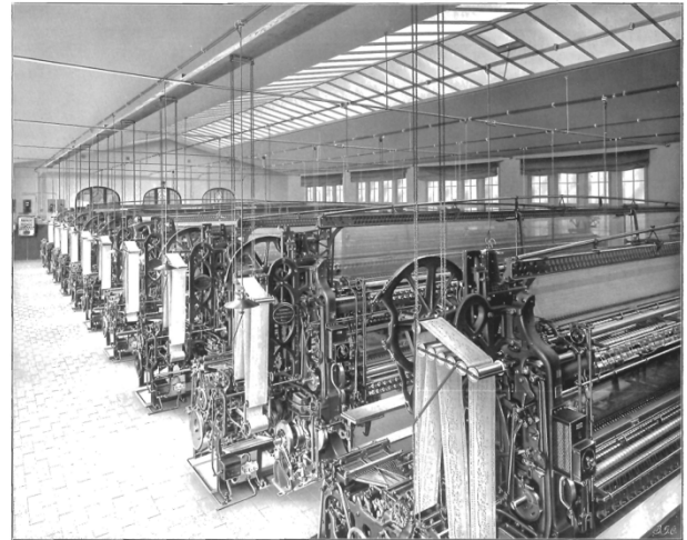
Abb. 19: Fabriksaal mit 10 Plauerer Schifflickstickmaschinen.
