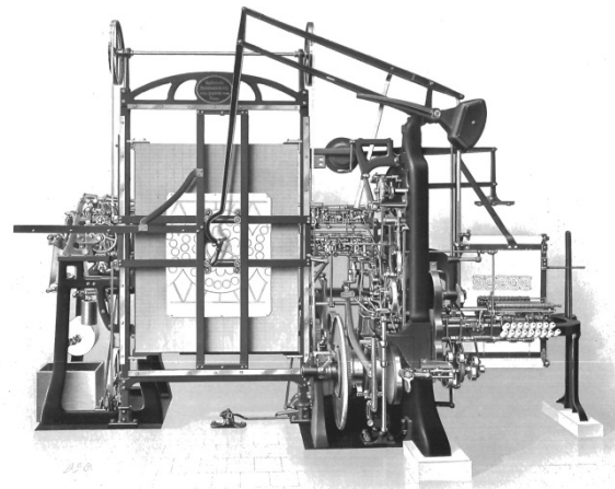
Abb. 20: Punchmaschine, System Zahn, Plauen.
