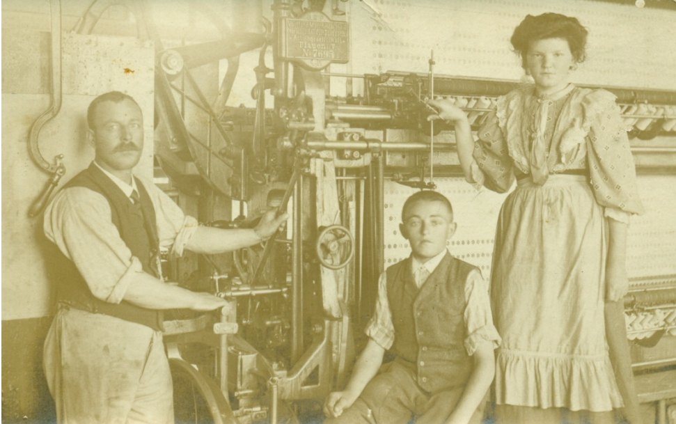
Abb. 11: Schifflistickmaschine mit Pantograph. Der Sticker führt die Maschine. Schifflifüller und Nachseherin sind Hilfskräfte. Aufnahme um 1900.
